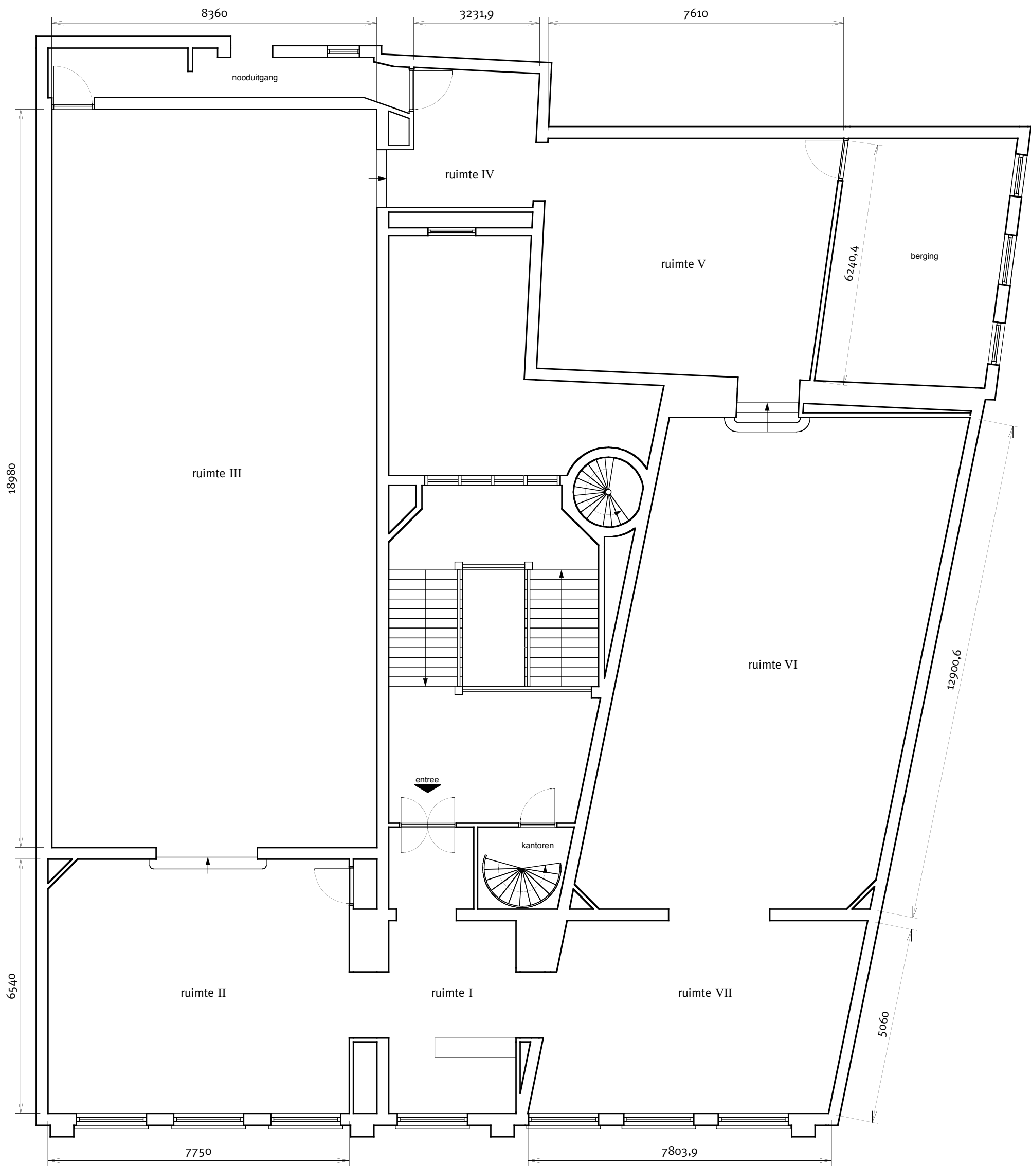
plattegrond Arti schaal 1:100
